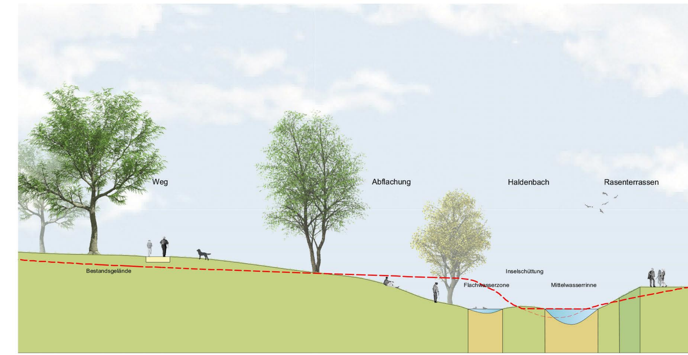
Schnitt BB Umbau / Renaturierung Haldenbach M 1:200
