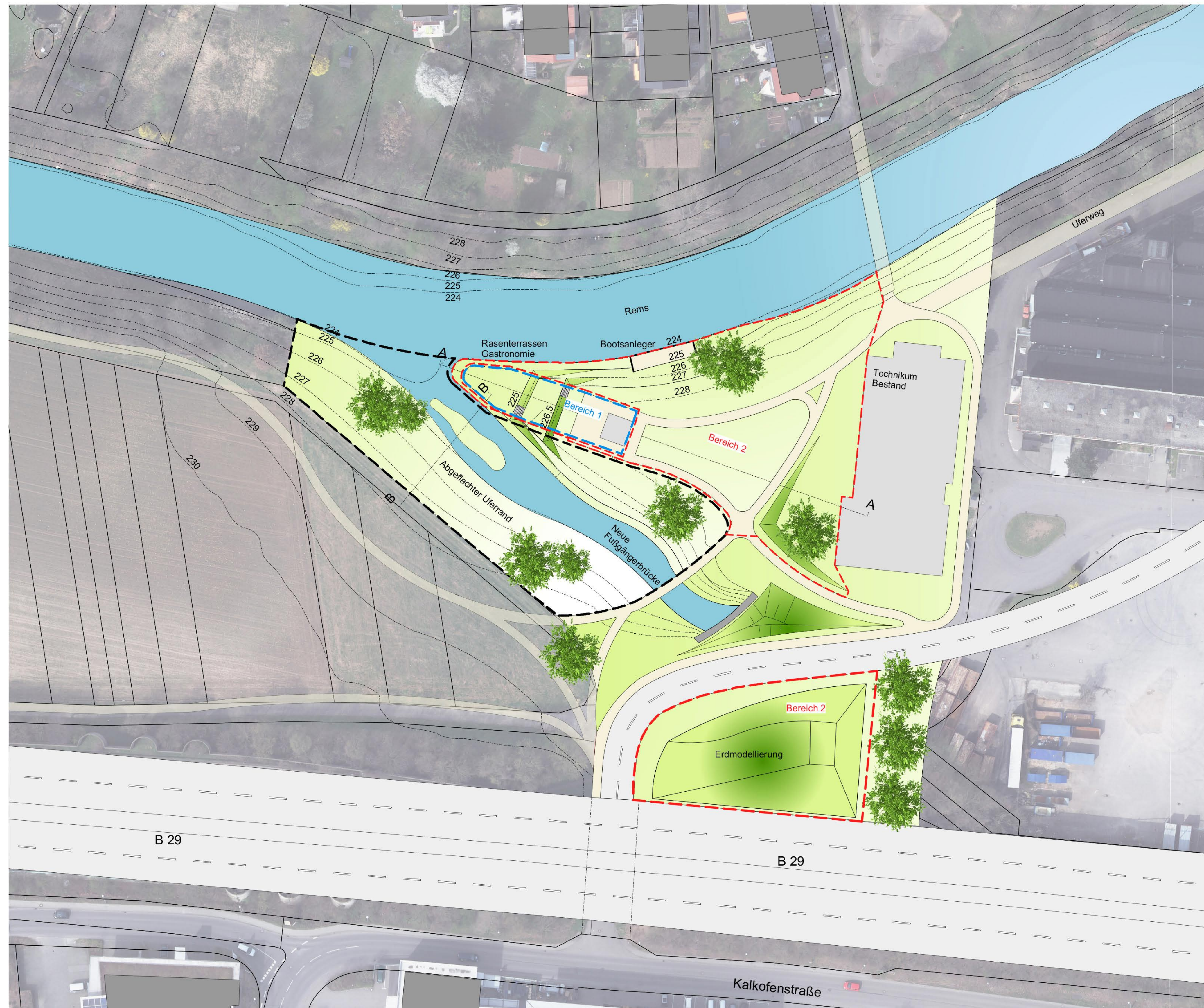
Lageplan M 1:500
