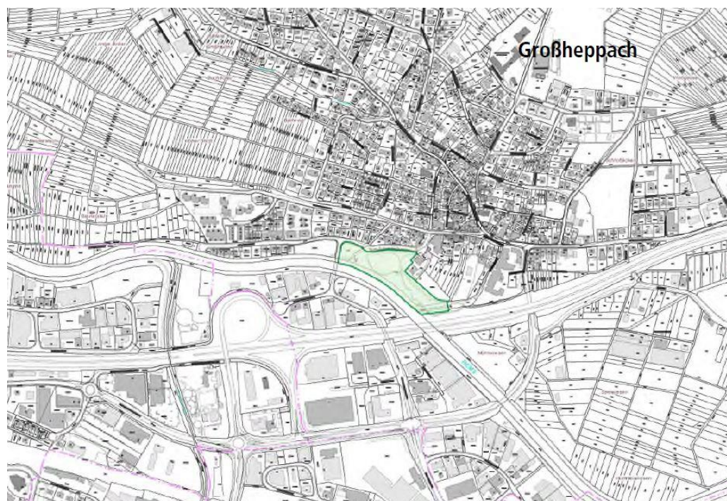
Abbildung 4.4: Lageplan der Maßnahme E3 Umgestaltung Mühlwiesen
