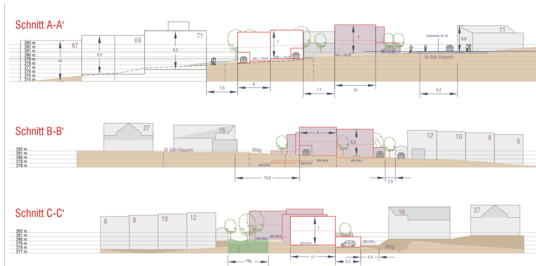
Abbildung 8: Schnittdarstellungen, Büro Baldauf, 06.05.2022
