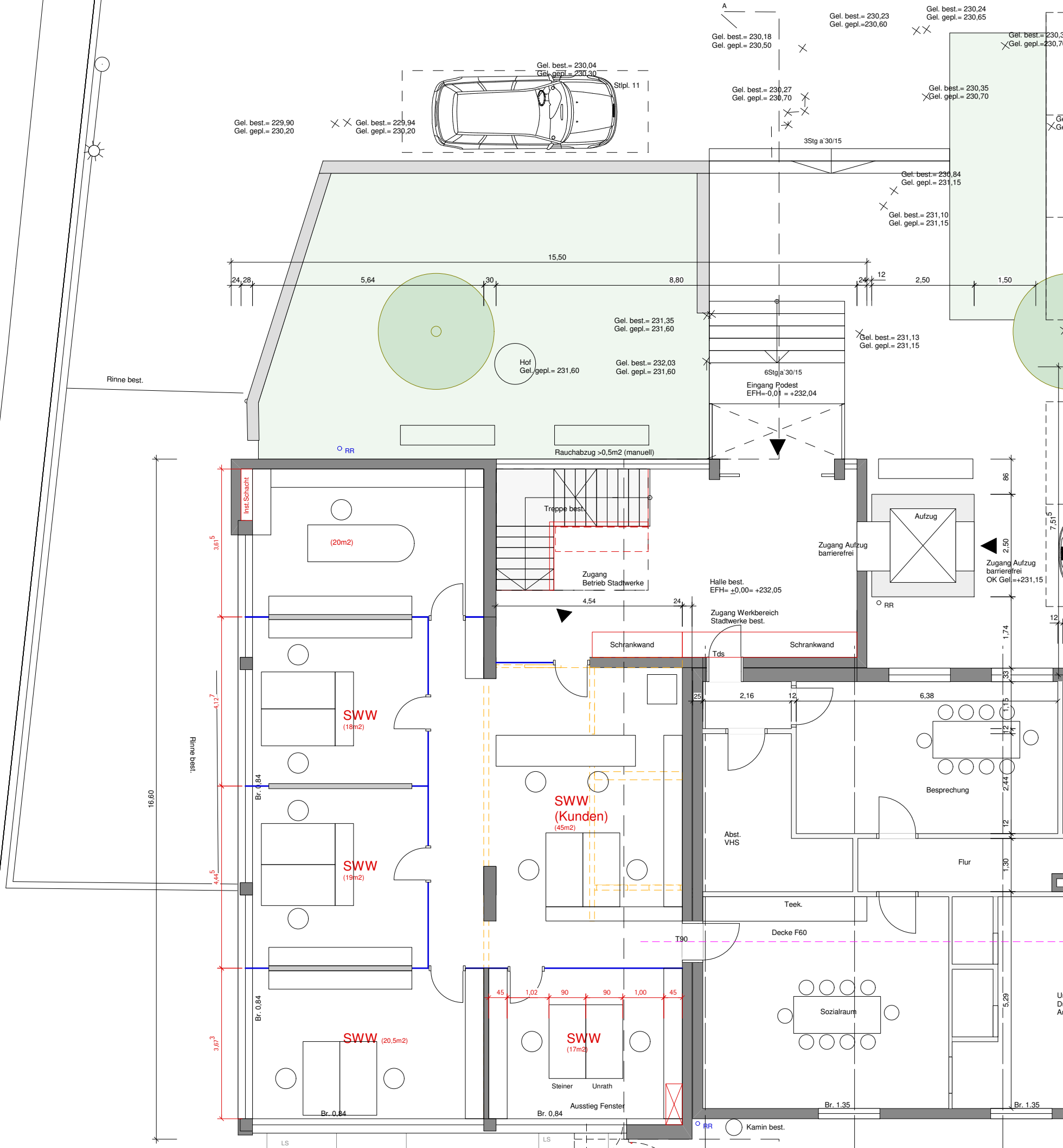
Erdgeschoss M 1/100 UMPLANUNG Weinstadt, 28.1.2018
