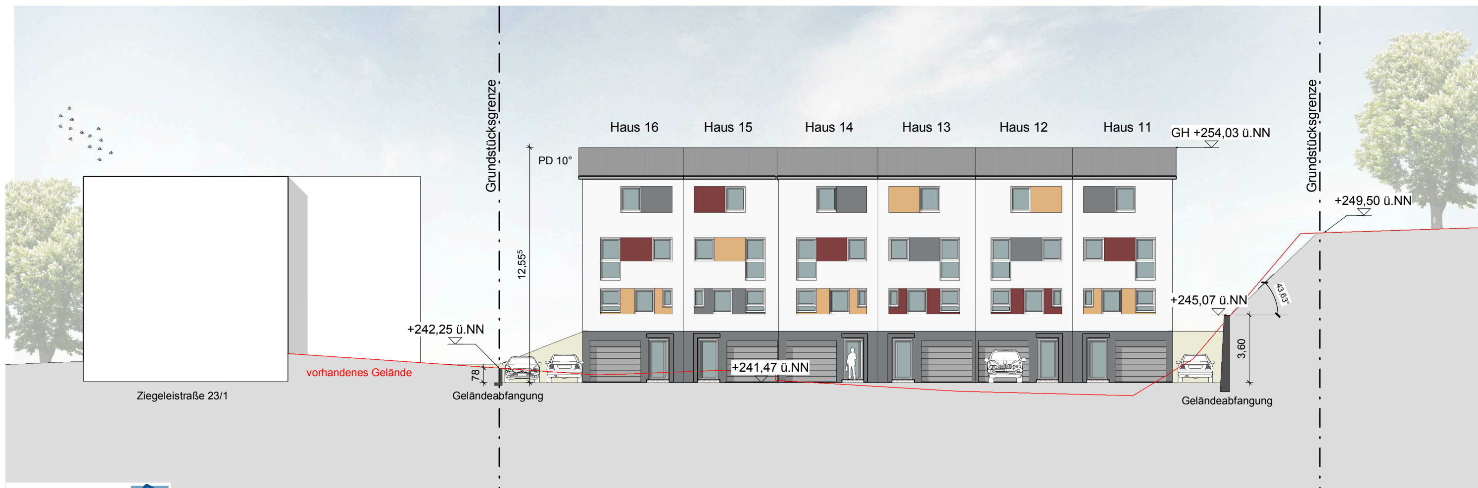
Ansicht Nord Haus 11-16
