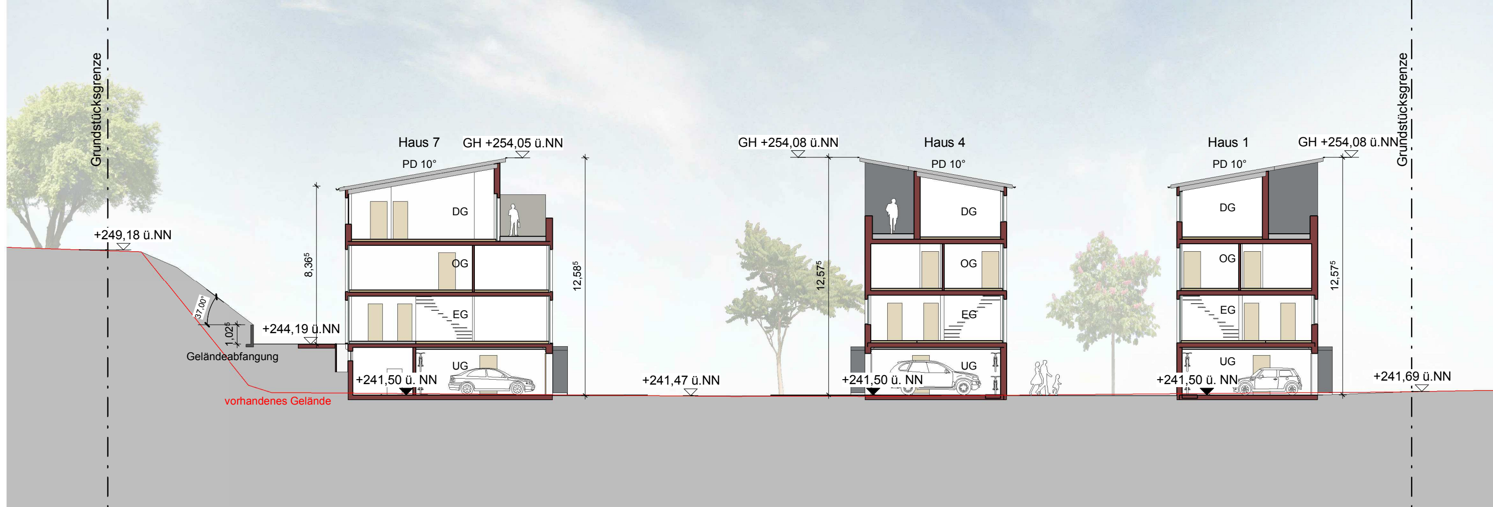
Schnitt 1
