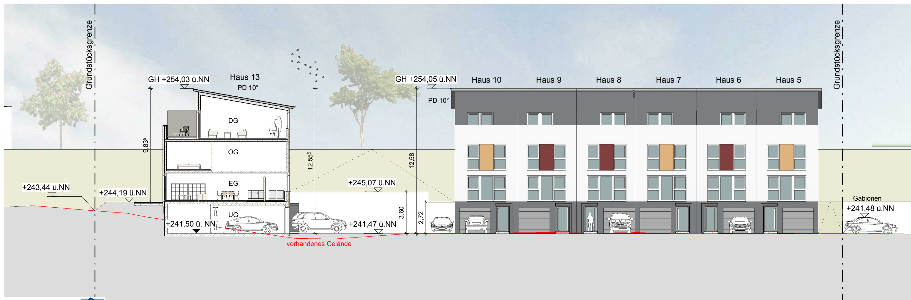
Ansicht Ost Haus 5-10
