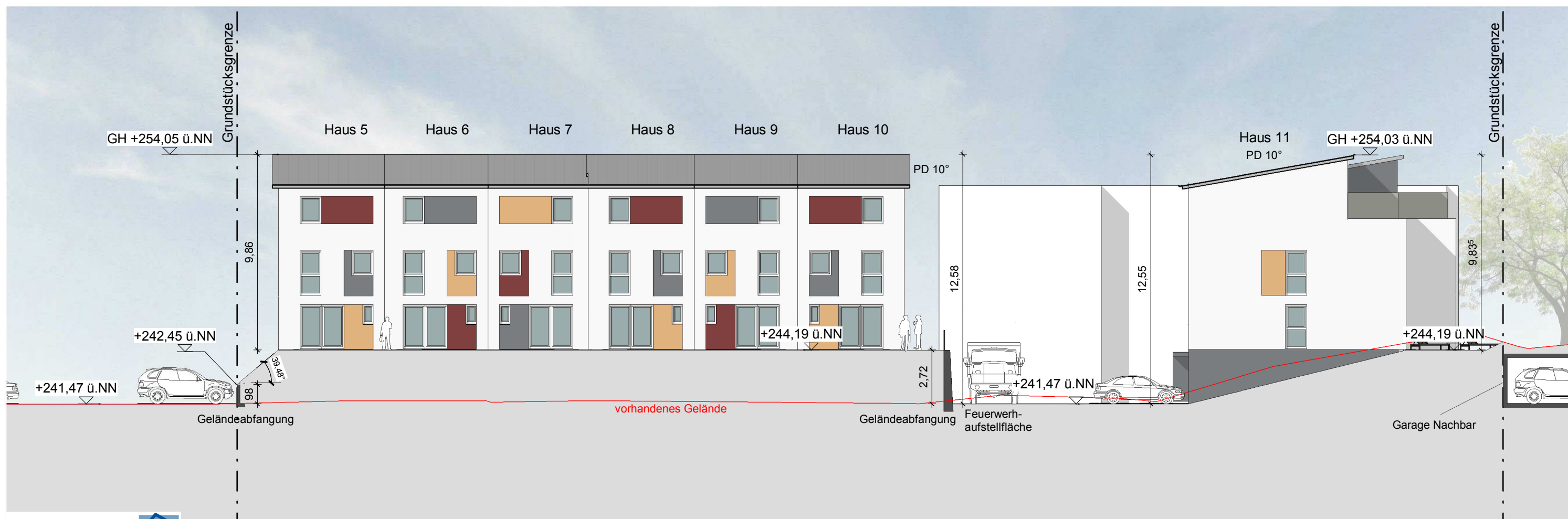
Ansicht West Haus 5-10 + 11
