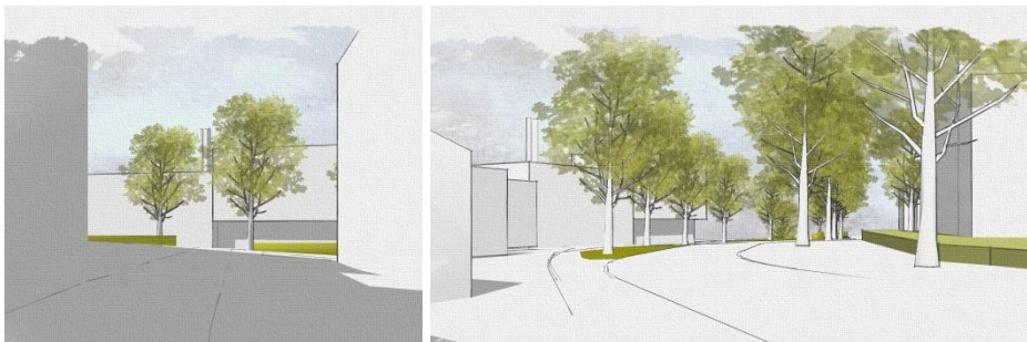
Abbildung 7: 3D-Modell des städtebaulichen Konzepts Endersbach West (Halde IV und Halde V), Baldauf Architekten und Stadtplaner GmbH, April 2017, Blick von Wohnweg zwischen Kornblumen und Lußackerweg (links), Blick von Süden aus der Metzgerackerstraße (rechts)
